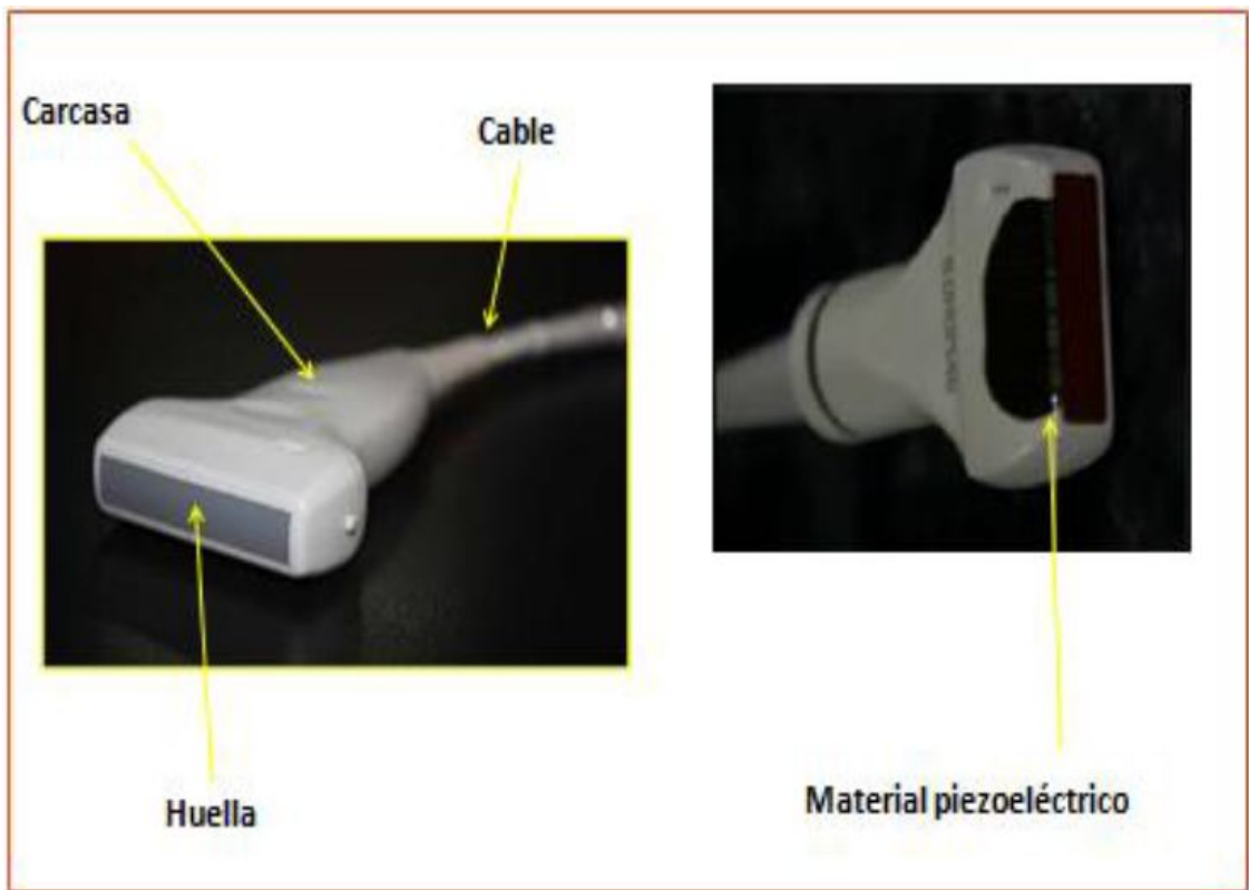
Figura 7. Componentes de una sonda ecográfica
